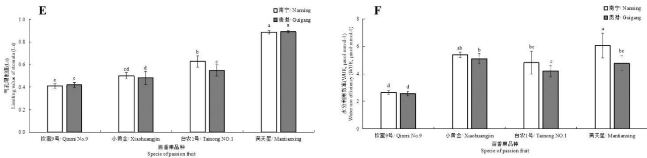
图4 持续高温条件下种植基地4个百香果品种光合特征参数
