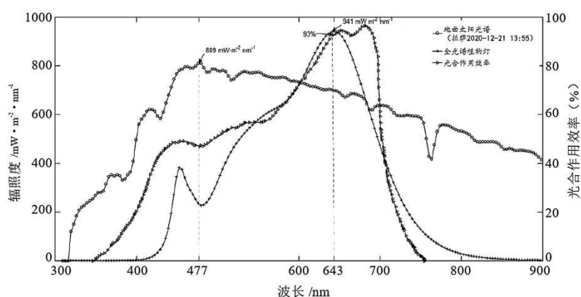
图 2 全光谱 LED 灯光谱
